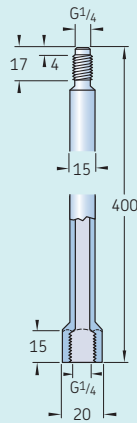
Tubo alargador de rosca G 1 / 4
